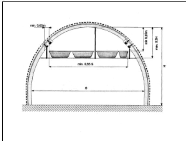
Figura C.19 Disposición de cubas de agua en una sección perpendicular de la galería de avance según la regulación polaca
