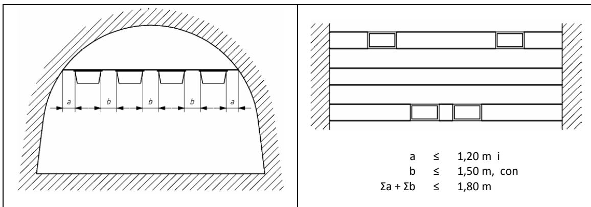
Figura C.4 Disposición de cubas de agua en la sección perpendicular. Distancias horizontales entre cubas
