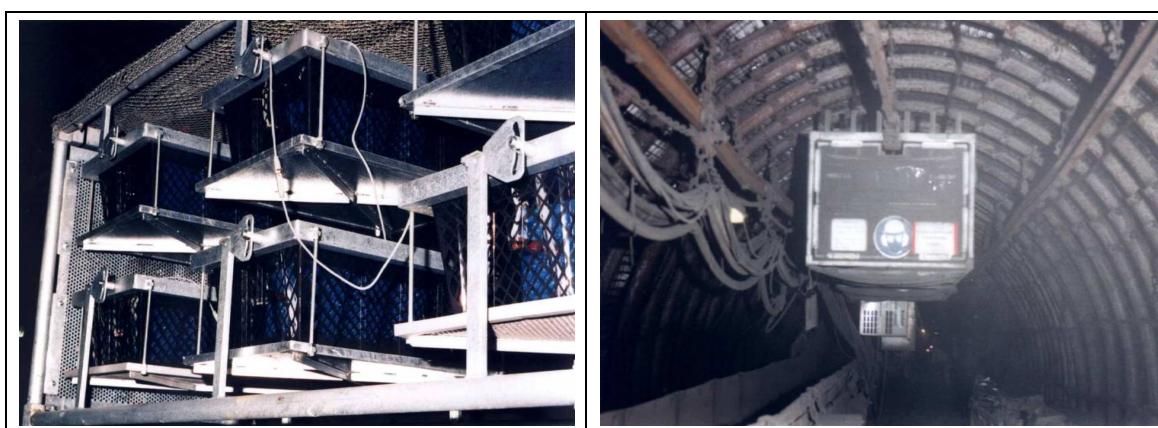
Fotografía C.2 Barrera activa de cubas de agua SaarEx 2000
