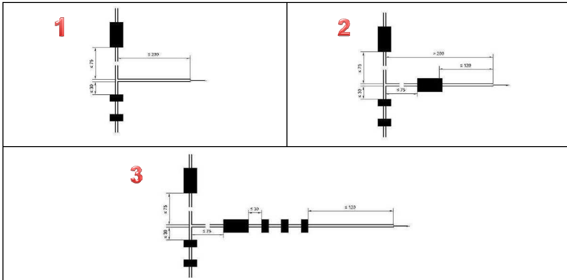
Figura C.18: Distancias entre barreras distribuidas en el avance de galerías con primera barrera concentrada
