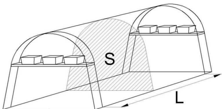
Possible disposición de una barrera distribuida ( L \leq 30 m)
