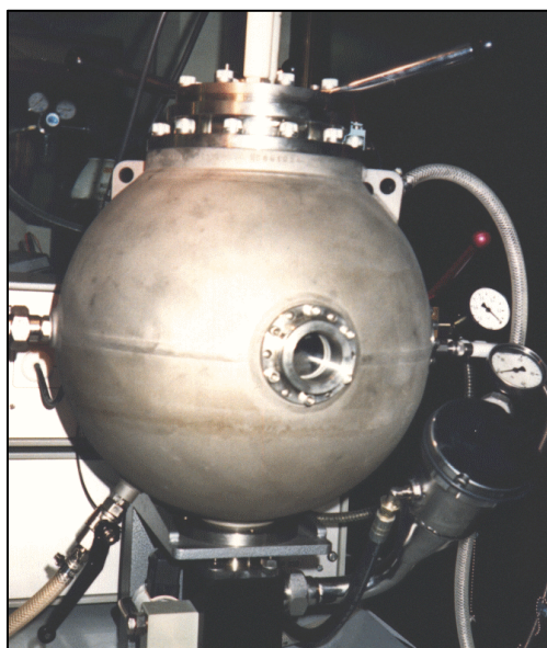
Fotografía A.3 Determinación de P_{max} y K_{max}
