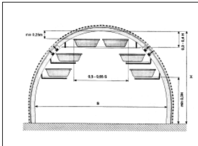
Figura C.20 Disposición lateral de cubas de agua en la sección perpendicular en la galería de avance según la regulación polaca
