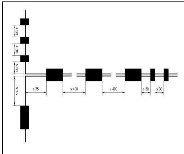
Figura C.15: Distancia para barreras de cubas de agua concentradas y distribuidas
