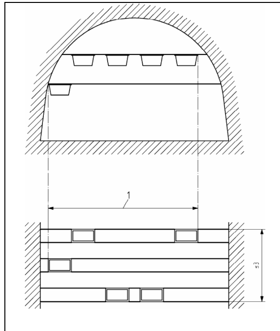
Figura C.5 Disposición de cubas de agua en la sección perpendicular. Distancia máxima horizontal de grupos
