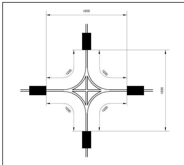
Figura C.13: Cordón de barreras para intersecciones de galerías con poca distancia entre ellas
