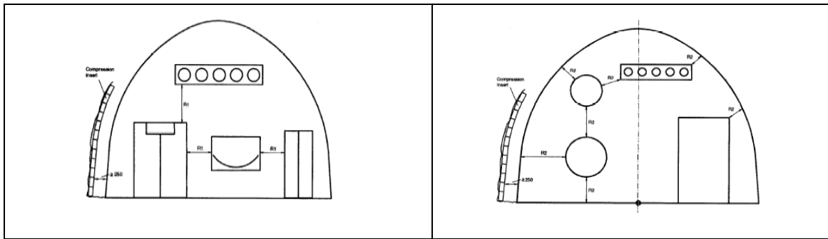
Figura C.24. Representación esquemática del espesor de las nervaduras R1 y R2 entre la puerta de transporte y la puerta de paso de personal y otras fijaciones.
