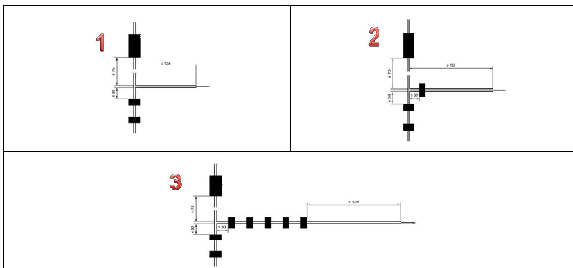
Figura C.17: Distancias entre barreras distribuidas en el avance de galerías
