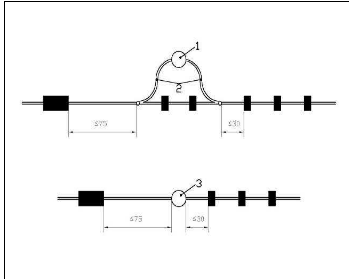
Figura C.12 Cordón de barreras en intersección de galerías con poca distancia entre ellas (1 – 3-Pozos verticales, 2- Galerías de acceso)
