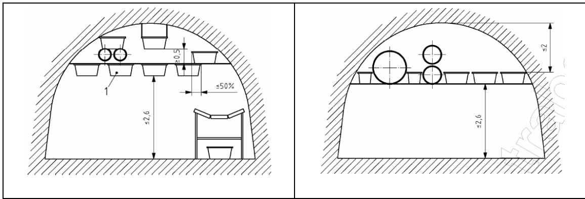
Figura C.3 Ubicación de las cubas de agua en una sección perpendicular de avance. Distancias verticales desde galería y entre cubas
