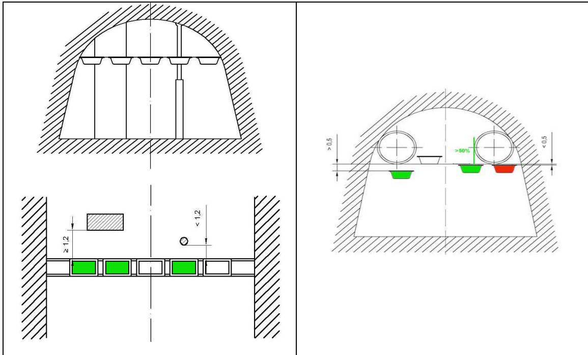
Figura C.7 Distancias a obstáculos
