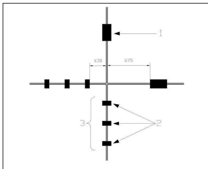
Figura C.11 Cordón de barreras en intersección de galerías
