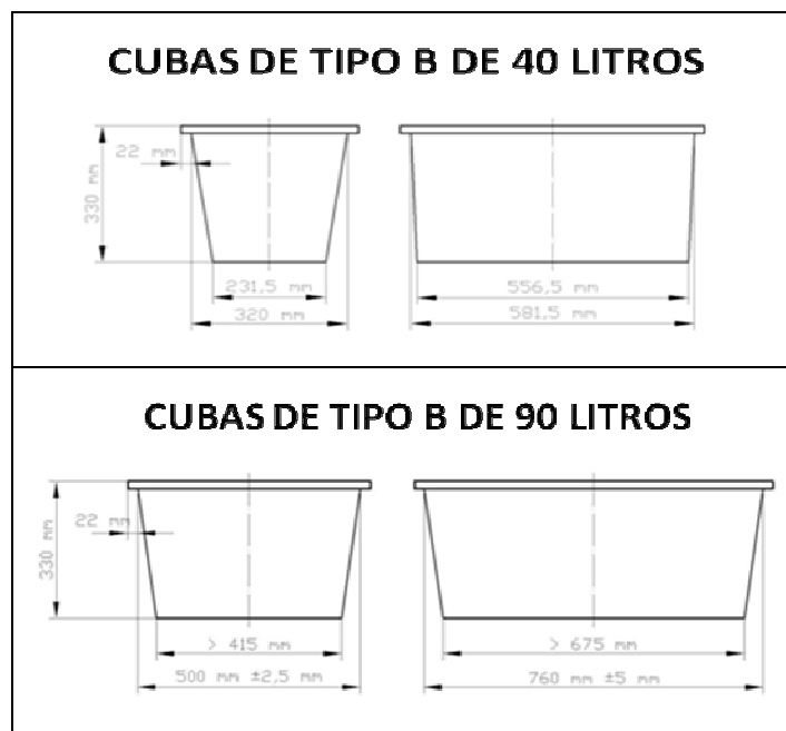
Figura C.10 Geometría de la cubas de tipo B para su instalación en estanterías
