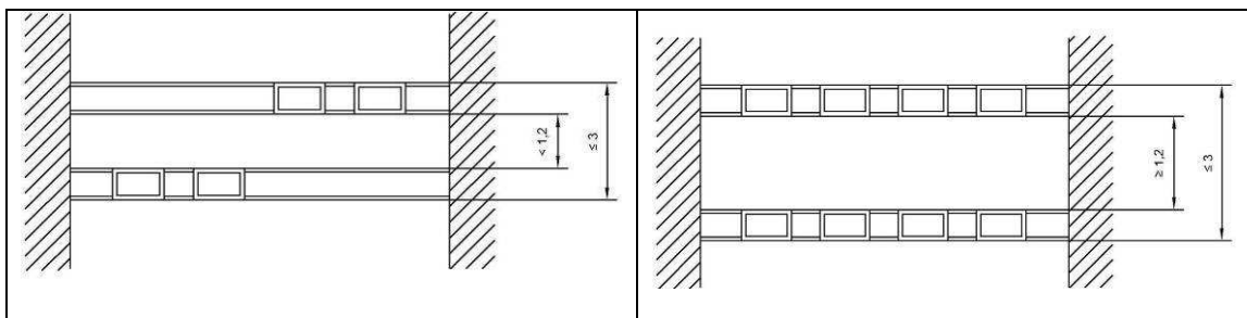
Figura C.8 Superposición entre filas de cubas de un grupo
