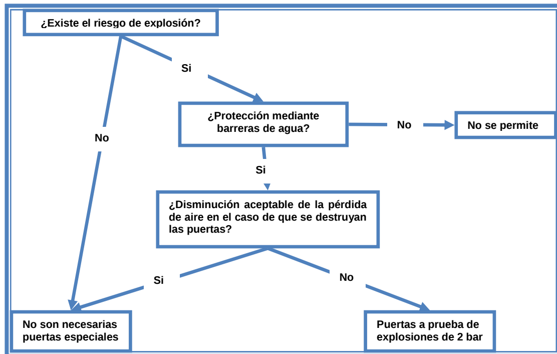
Figura C.23 Diagrama de decisión para la instalación de barreras de protección contra explosiones
