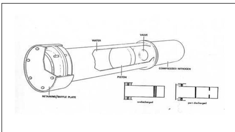
Figura C.21 Barrera de cilindro diseñada por el SMRE
