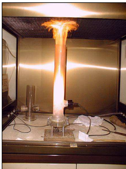
Fotografía A.2 Tubo del Hartmann
