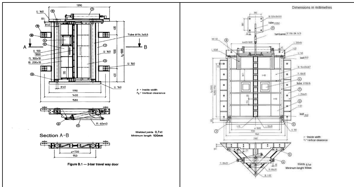
Figura C.25. Puertas de ventilación a prueba de explosión
