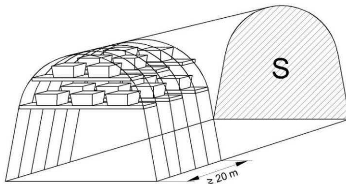
Possible disposición de una barrera concentrada
