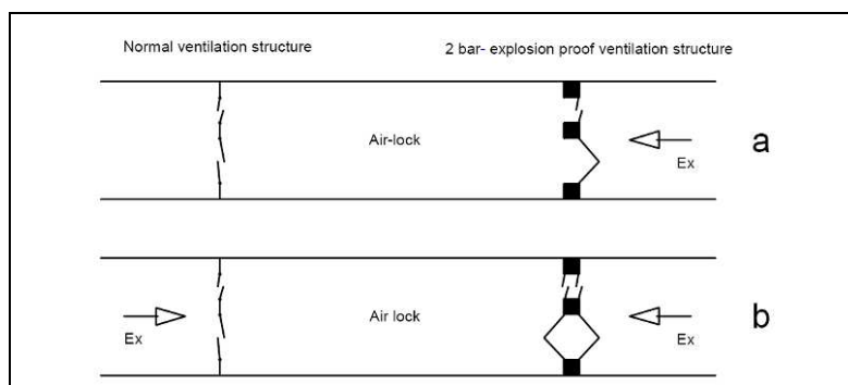
Figura C.26 Esquema de una estructura de ventilación a prueba de explosiones
