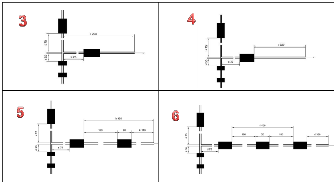
Figura C.16: Distancias entre barreras concentradas en el avance de galerías
