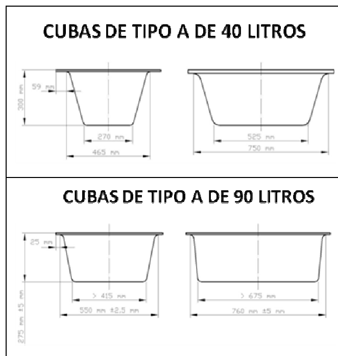
Figura C.9 Geometría de la cubas de tipo A para su instalación en bastidores
