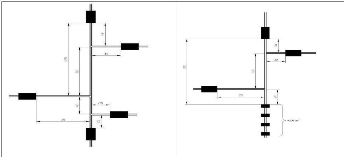
Figura C.14: Cordón de barreras para entronques con poca distancia entre ellos
